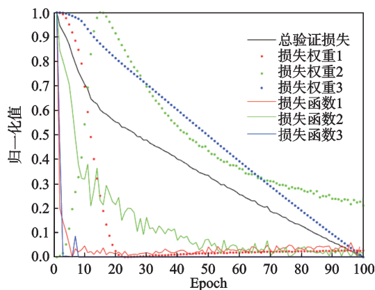
图11 不确定性损失权重平衡迭代过程
