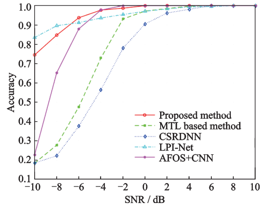
图 16 不同模型实验效果对比
