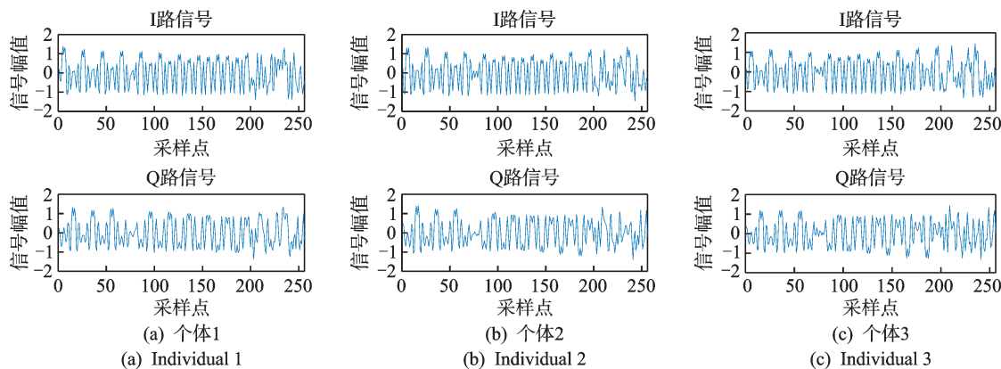
图7 3个不同个体IQ信号波形
