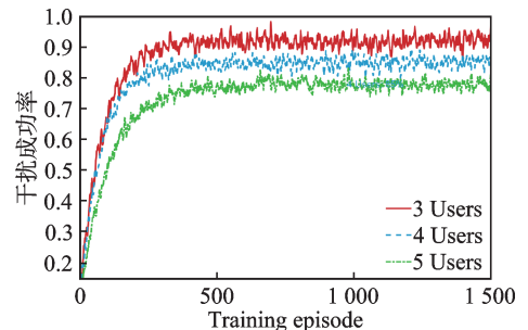
图9 不同用户干扰成功率对比曲线
