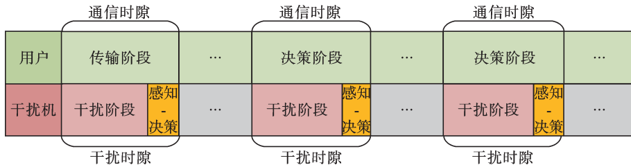
图3 干扰-用户时隙结构
