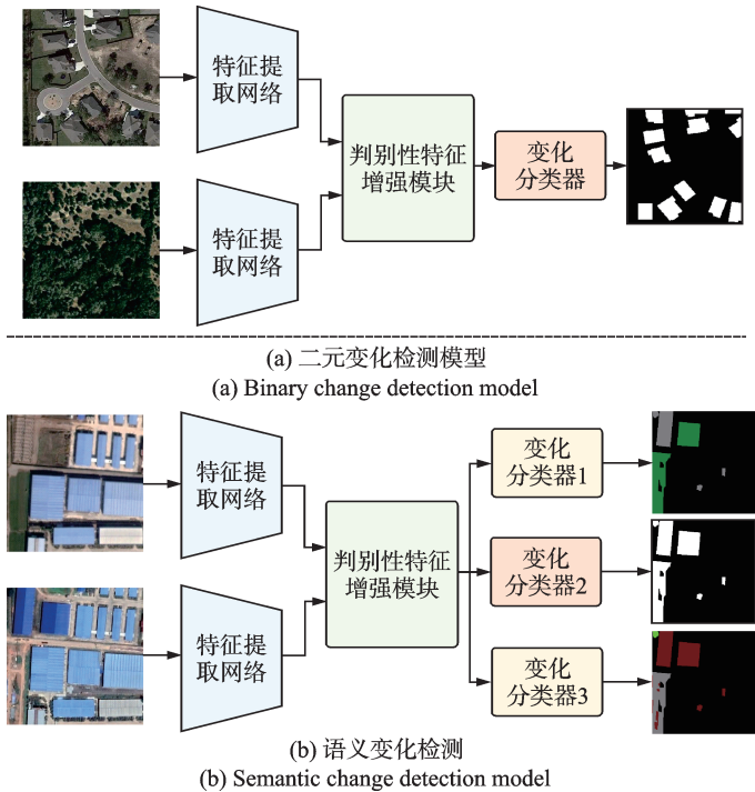
图2 二元和语义变化检测典型模型
