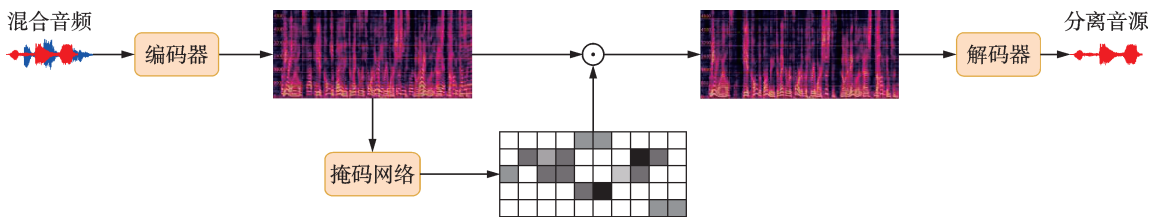
图2 基于时频掩码的音源分离系统框图 [23]
