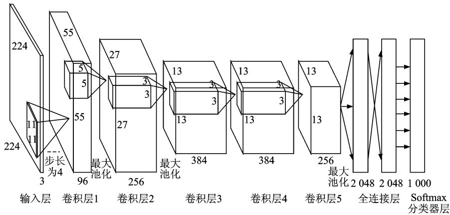
图 4 简化的 AlexNet 模型结构 Fig. 4 Simplified structure of AlexNet model
