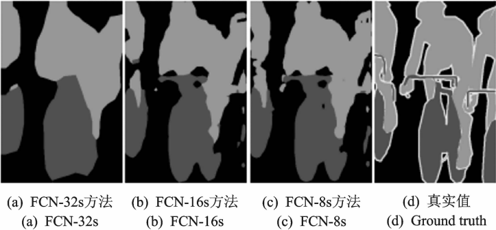
图 17 各种方法结果的比较 [35] Fig. 17 Results of different methods [35]
