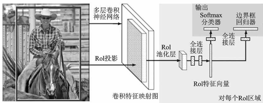
图 9 Fast R-CNN 结构示意图 [31] Fig. 9 Fast R-CNN architecture [31]
