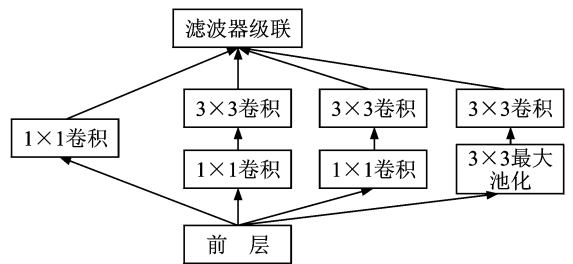
图 5 简化的 Inception 模块结构 [20] Fig. 5 Simplified structure of Inception module [20]
