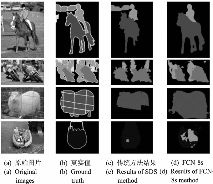
图 18 FCN,SDS 在 PASCAL VOC 上的一些结果 [35] Fig. 18 Some results given by FCN and SDS on PASCAL VOC [35]
