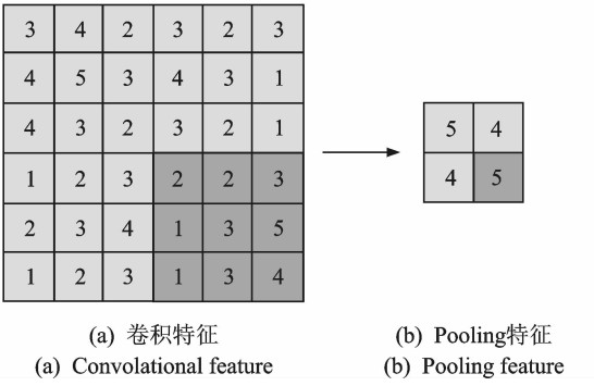
图 3 最大池化运算操作示意图 Fig. 3 Illustration of max pooling operation
