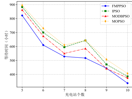
(b) 等待时间目标随站点个数变化
