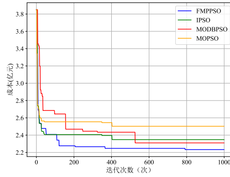
(d) 不同算法的收敛曲线
