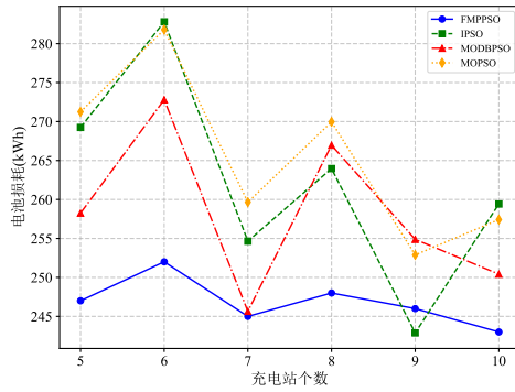
(c) 电池损耗目标随站点个数变化
