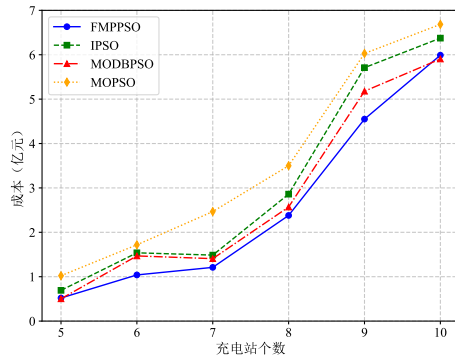
(a) 成本目标随站点个数变化
