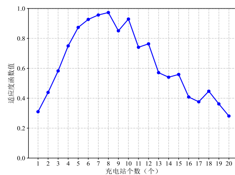
图 4 FMPPSO 适应度函数变化 Fig.4 Changes in FMPPSO fitness function
