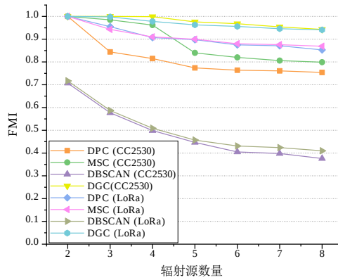
图 7 辐射源数量变化时不同算法识别性能
