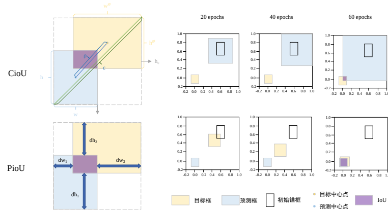
图 5 CIoU 和 PIoU 的锚框变化图
