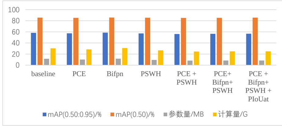
图 6 消融实验指标对比
