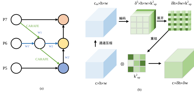
图 3 Bifpn 结构 (a) 和 CARAFE (B)
