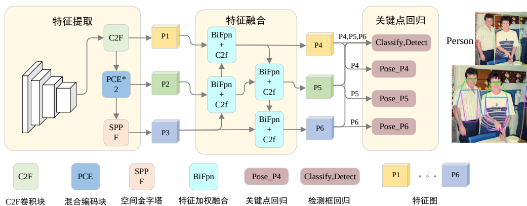
图 1 PCE_LitePose 模型结构
