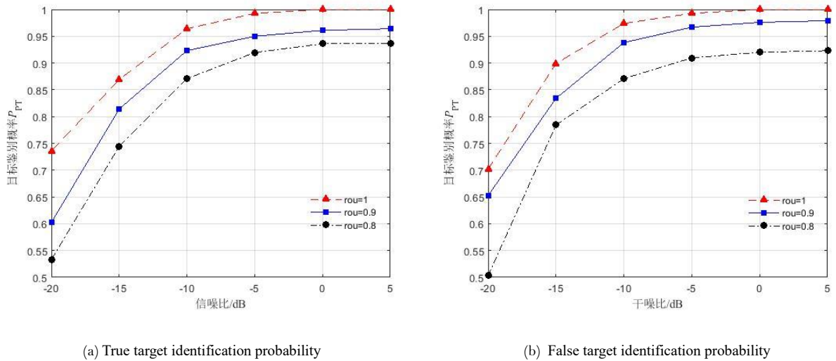
图 6 相位同步对目标鉴别概率的影响
