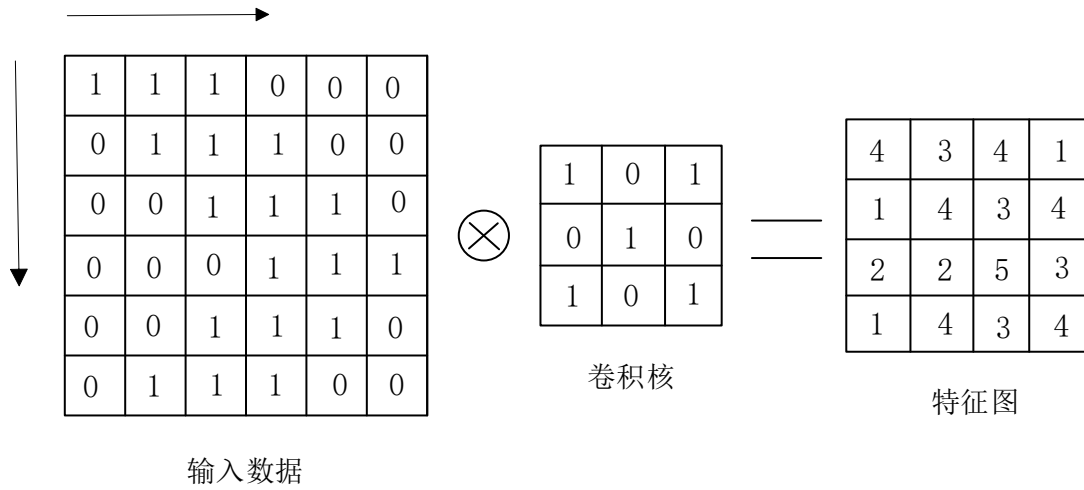
图 2 卷积层过程
