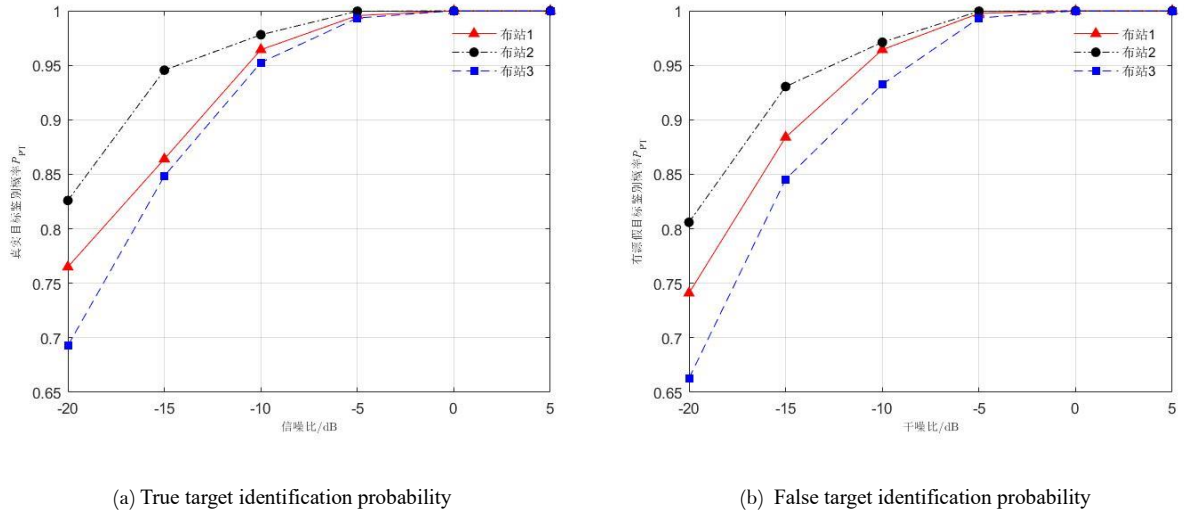
图 5 不同布站情况下目标鉴别概率
