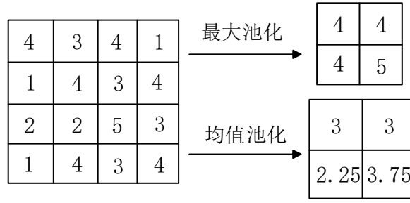
图 3 池化层过程
