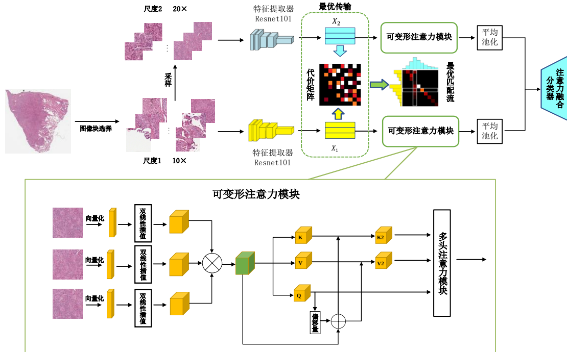
图 1 DMSMIL 的总体框架
