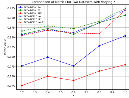
图 3 不同 \lambda 在 TCGA-BRCA、TCGA-NSCLC 上结果图
