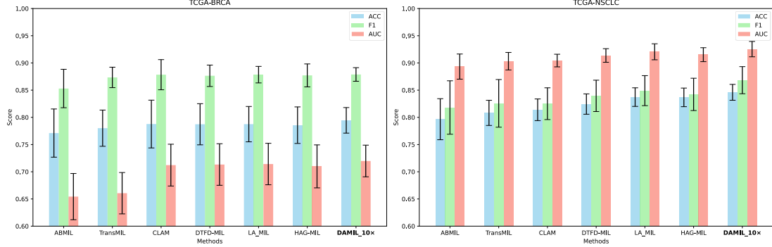
图 4 单尺度方法在 TCGA-BRCA、TCGA-NSCLC 数据集 10\times 尺度上对比实验结果
