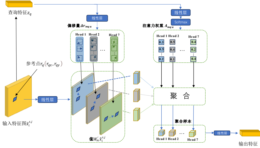
图2 可变形注意力模块
