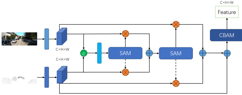
图 2 迭代深度感知注意力融合模块
