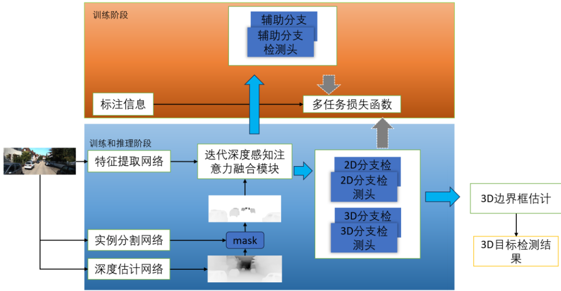
图 1 网络结构图
