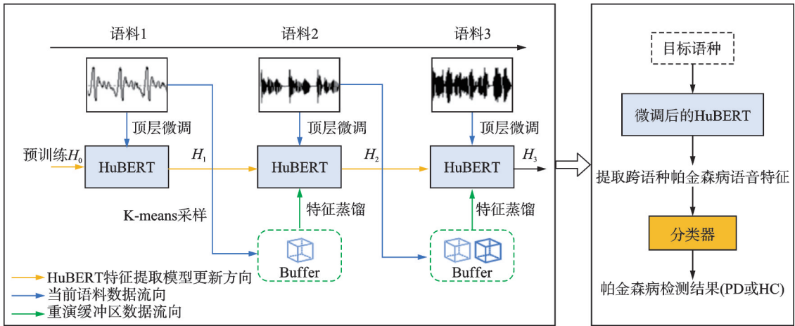
图1 持续自监督的跨语种帕金森病检测模型
