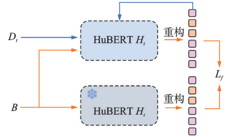
图4 特征蒸馏过程
