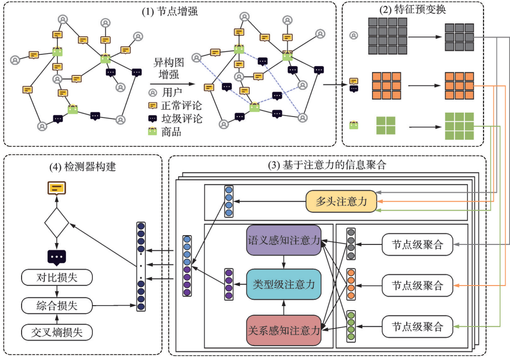
图1 基于神经网络的垃圾信息检测方法框架
