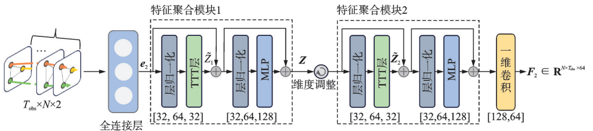
图4 时空交互模块
