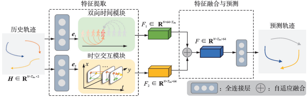
图1 模型整体结构
