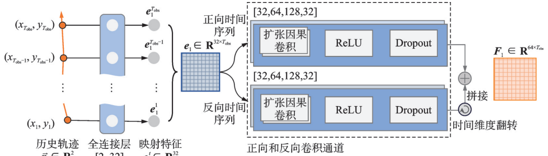
图2 时间依赖模块
