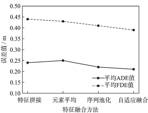
图5 不同融合方法对比
