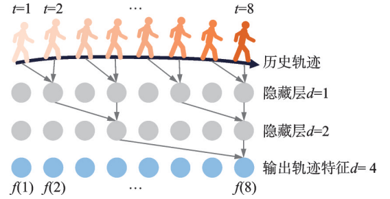
图3 扩张因果卷积示意图
