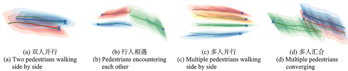
图 6 多模态轨迹预测分布可视化
