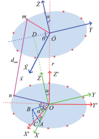
图1 非理想情况下发射端UCA和接收端UCA几何模型图
