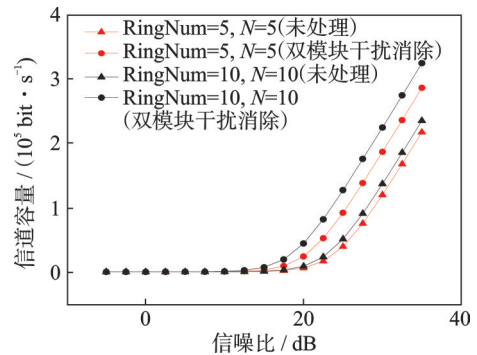
图5 双模块干扰消除方案处理与未处理的信道容量比较图
