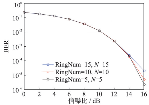
图4 不同UCA数量的BER比较图
