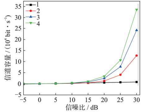
图3 不同UCA个数的信道容量比较图
