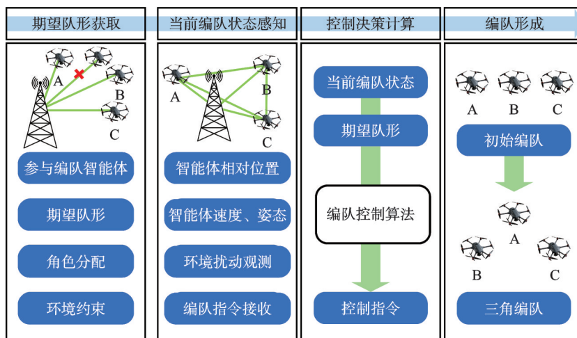
图 11 编队控制流程
