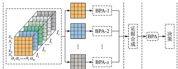
图3 基于D-S证据理论的多源信息系统的融合过程
